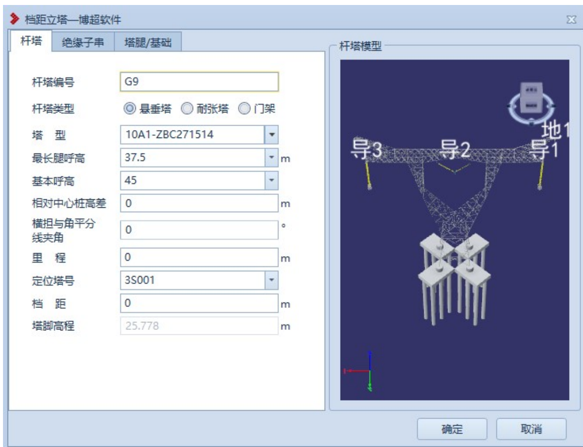
图 7.2- 28 档距立塔界面
