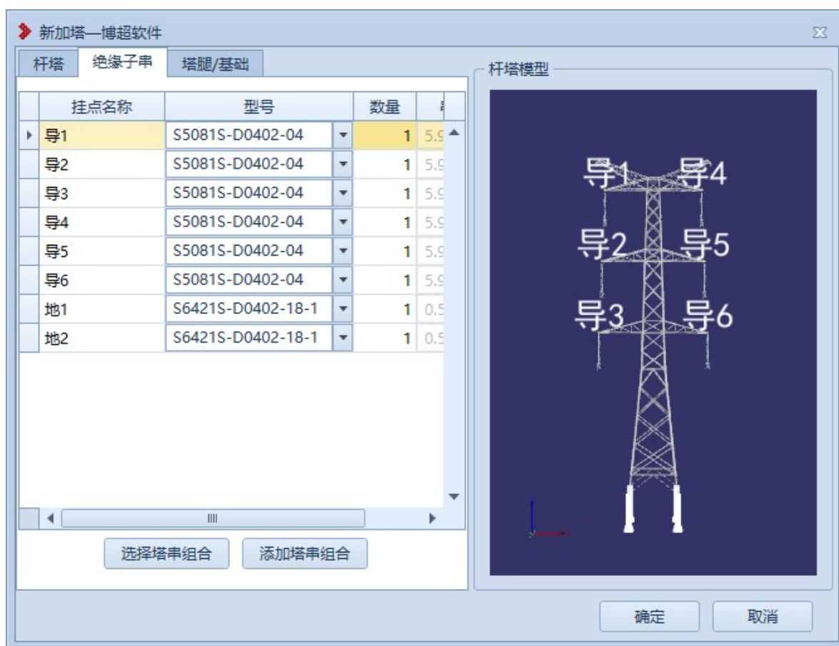
图 7.2- 25 新加塔-绝缘子串
