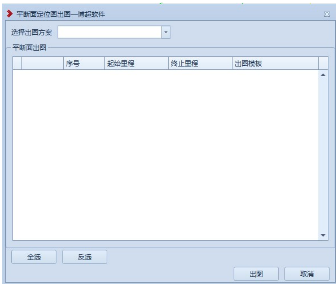
图 7.2- 57 平断面出图
