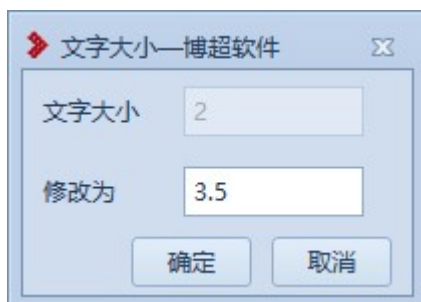
图 7.2- 70 文字大小
