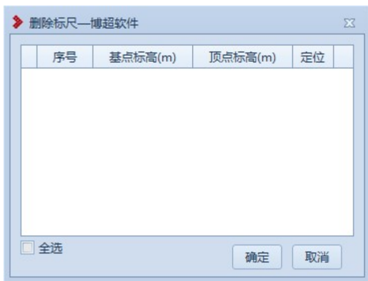
图 7.2- 17 删除标尺
