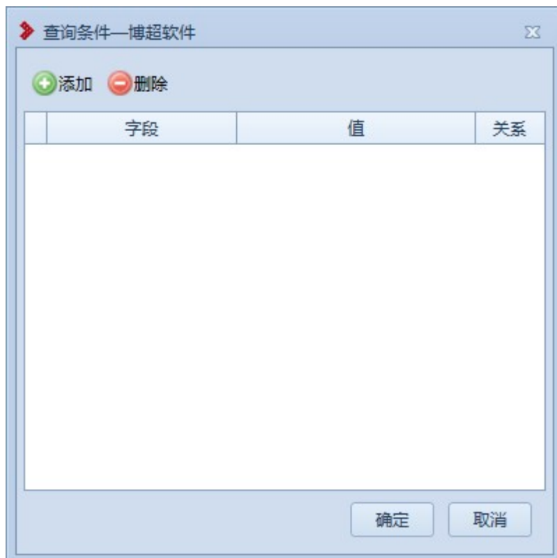
图 7.2- 23 查询条件
