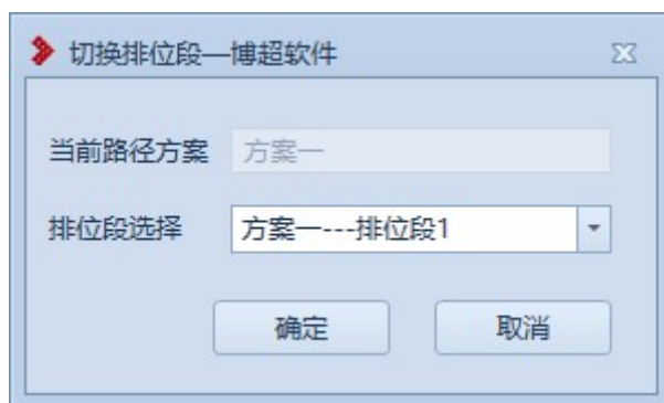
图 7.2- 1 切换排位段
