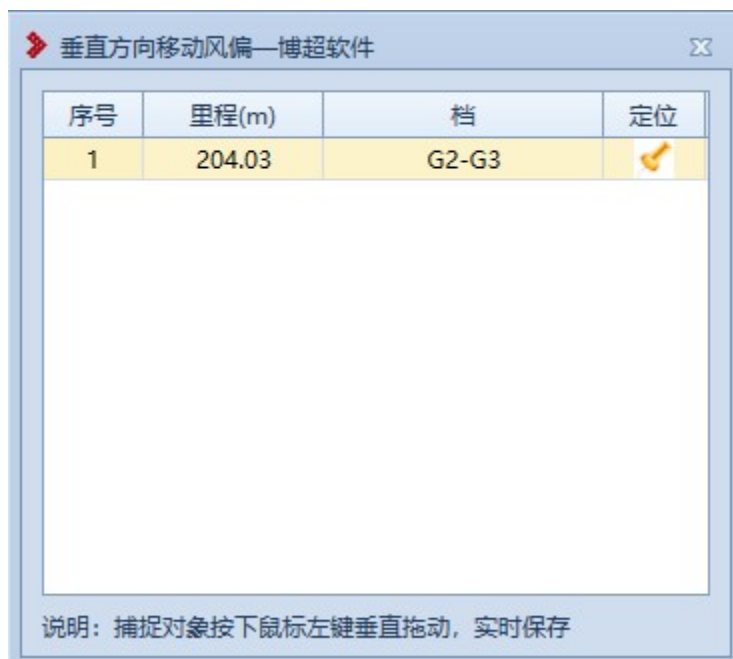
图 7.2- 48 移动风偏
