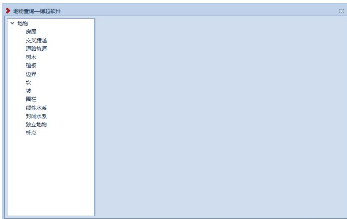
图 7.2- 21 地物查询
