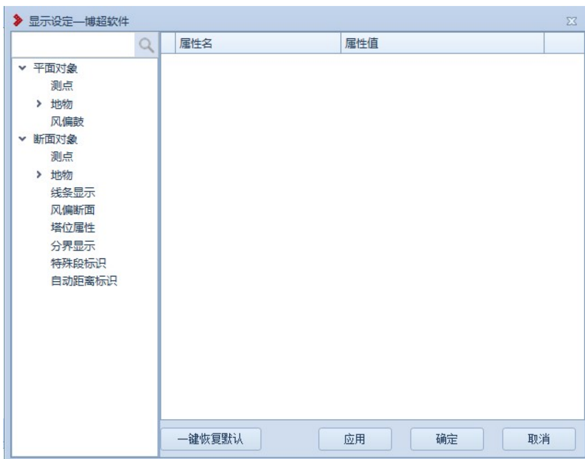
图 7.2- 69 显示设定
