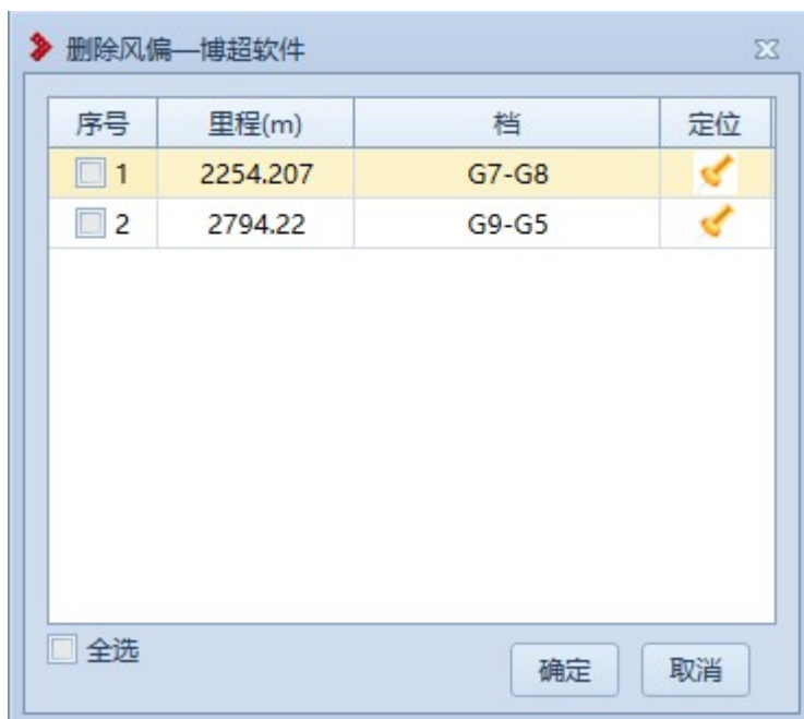
图 7.2- 47 删除风偏
