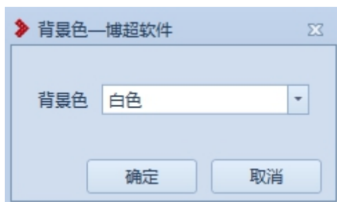
图 7.2- 72 背景色
