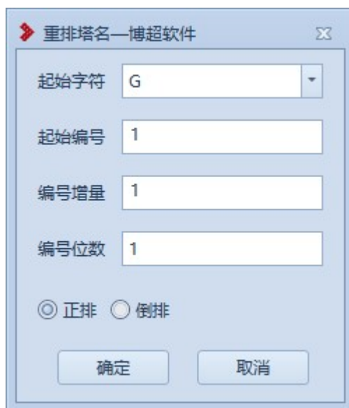
图 7.2- 36 杆塔编号
