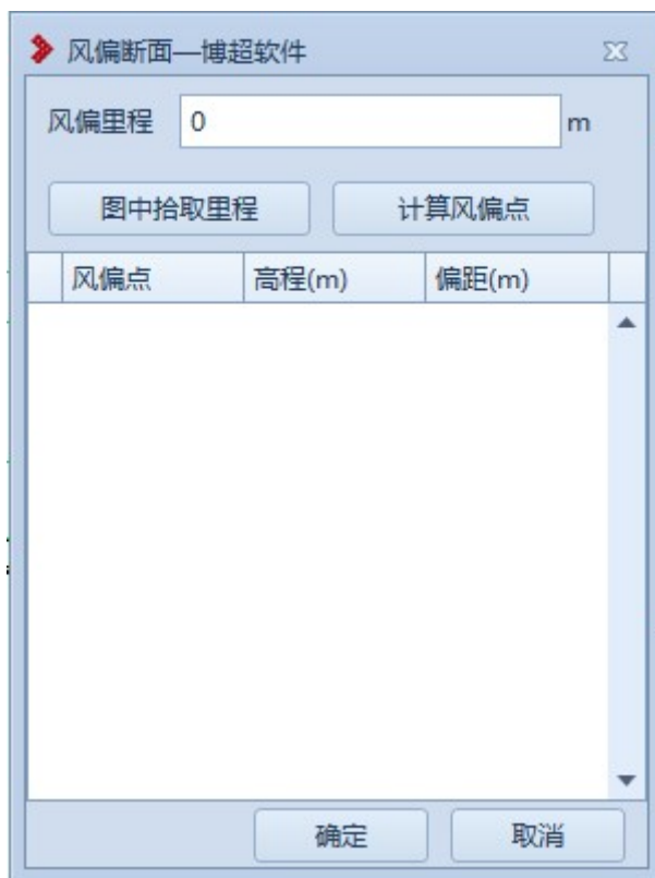
图 7.2- 45 风偏断面
