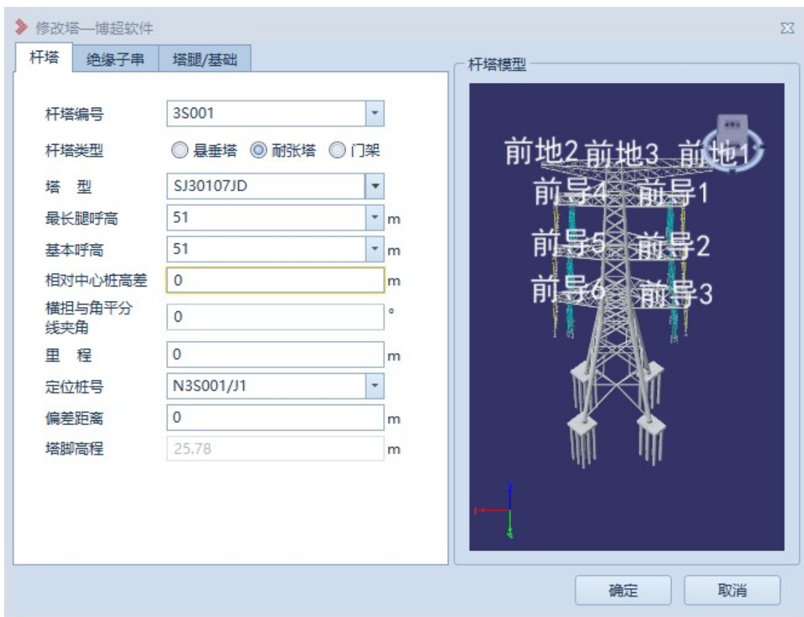
图 7.2- 29 修改塔-杆塔
