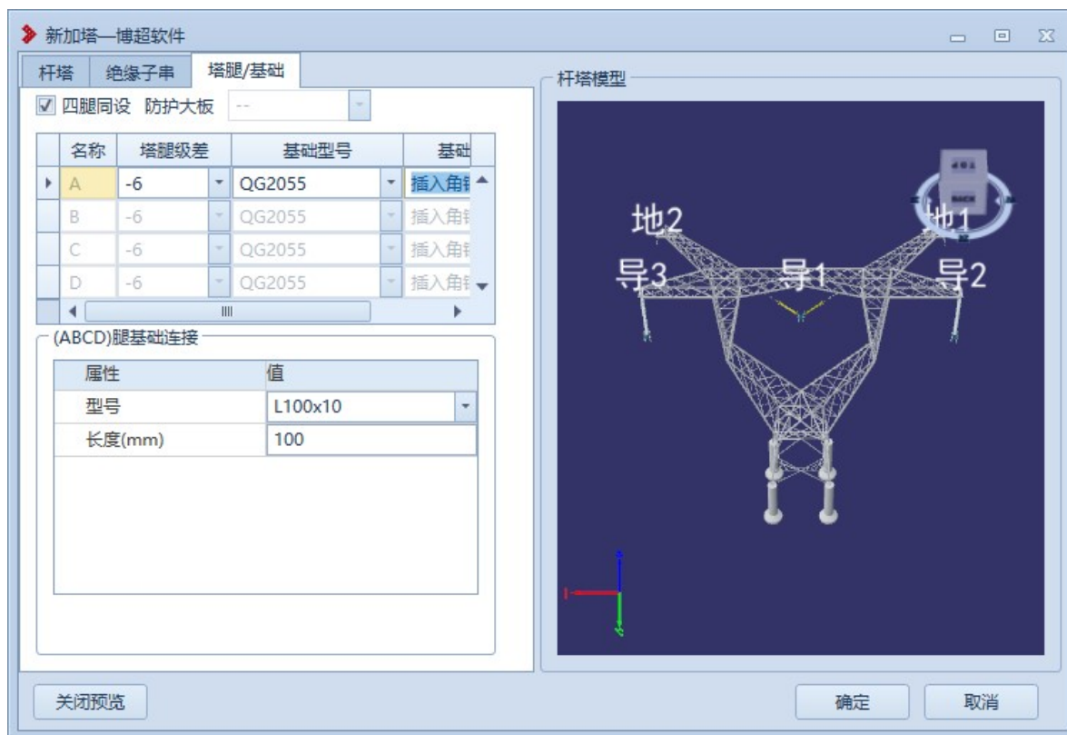
图 7.2- 28 新加塔-塔腿/基础-插入角钢
